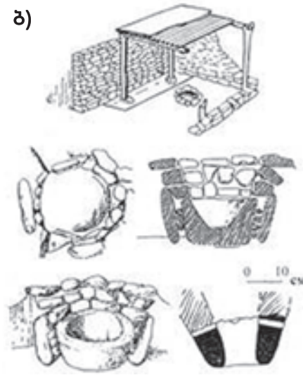
სურ. 3. ა) ლითონის ჩამოსასხმელი თიხის ფორმაები. (საქართველოს სახელმწიფო მუზეუმი). ბ) მეტალურგიული ცენტრი ამირანის ბორა. გ) ქურაში ჭანგბადის მისანოდებალი თიხის მილი მაღალი ტემპერატურის შესანარჩუნებლად.
